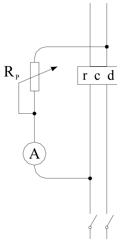
Αποσυνδεδεμένο φορτίο
