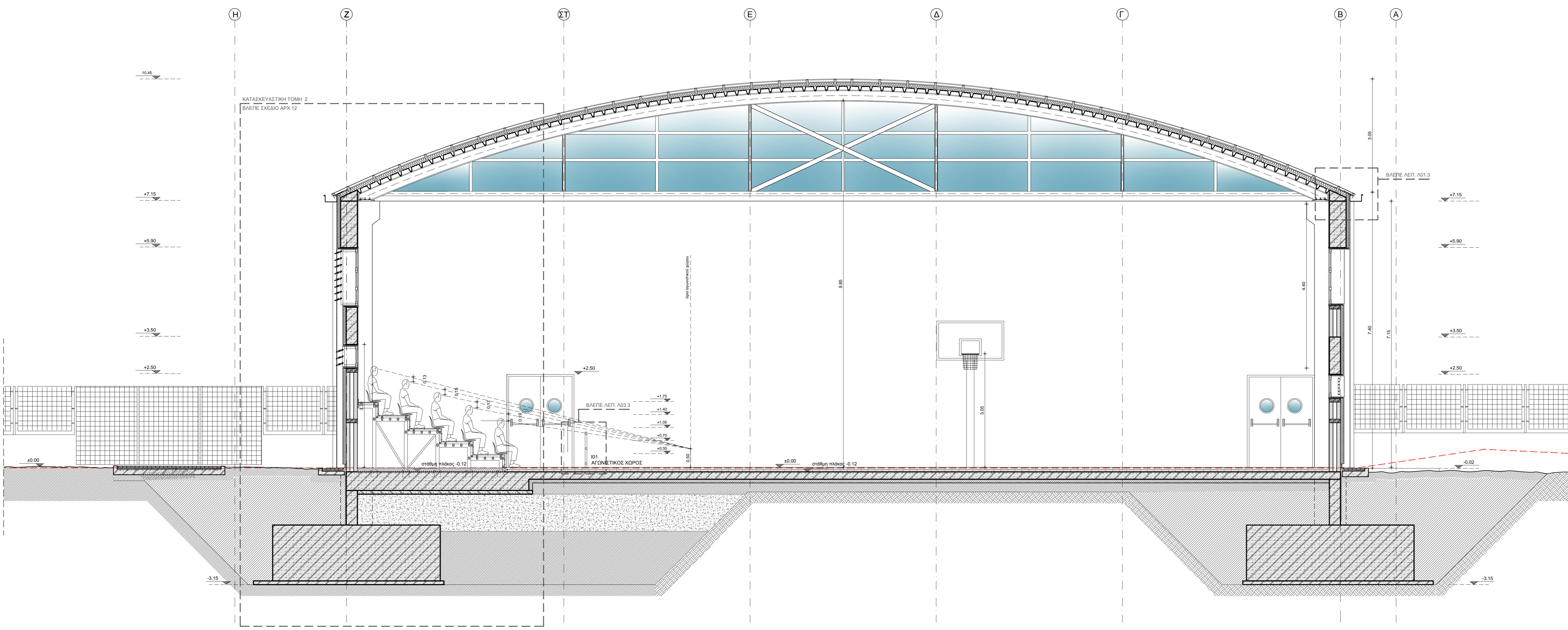
ΤΟΜΗ Γ - Γ'
