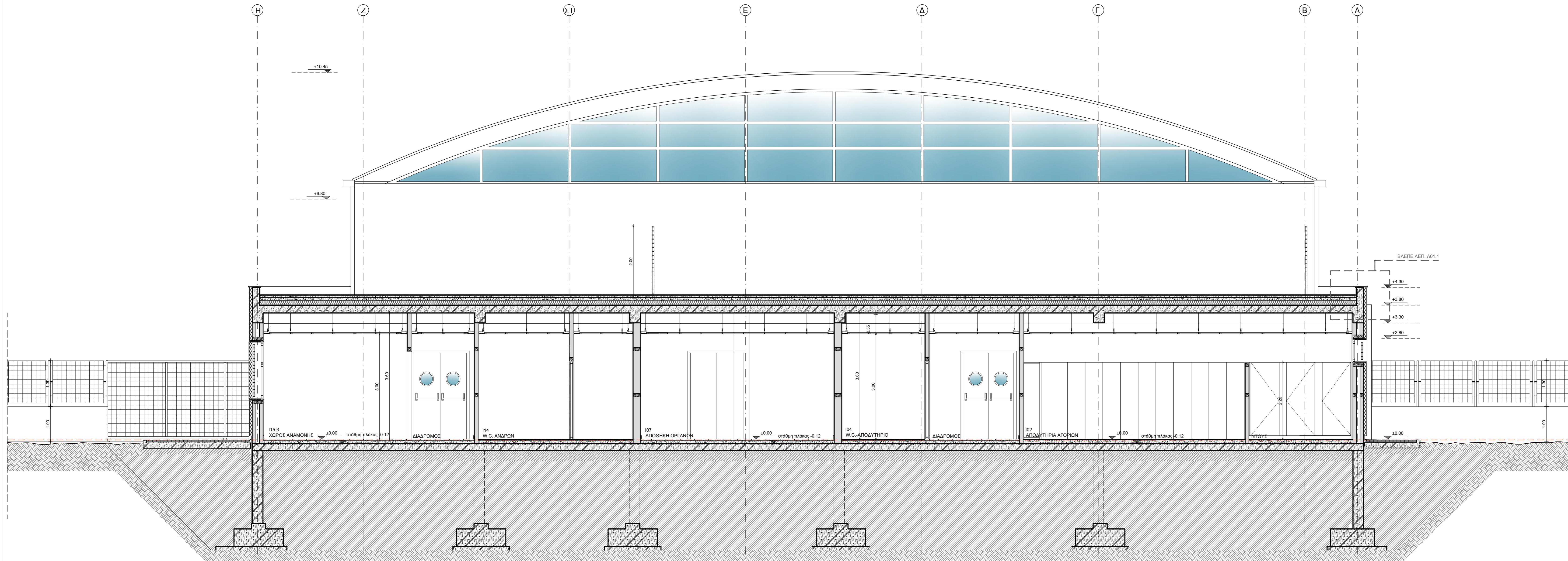
TOMH E - E'
