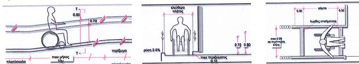
Τομή T-T
