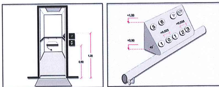
Χειριστήρια Ανελκυστήρων
